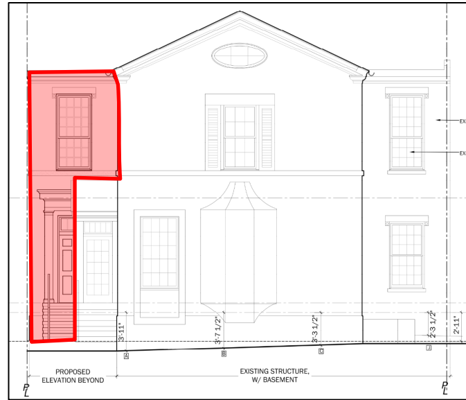
N. Alfred Street Façade
