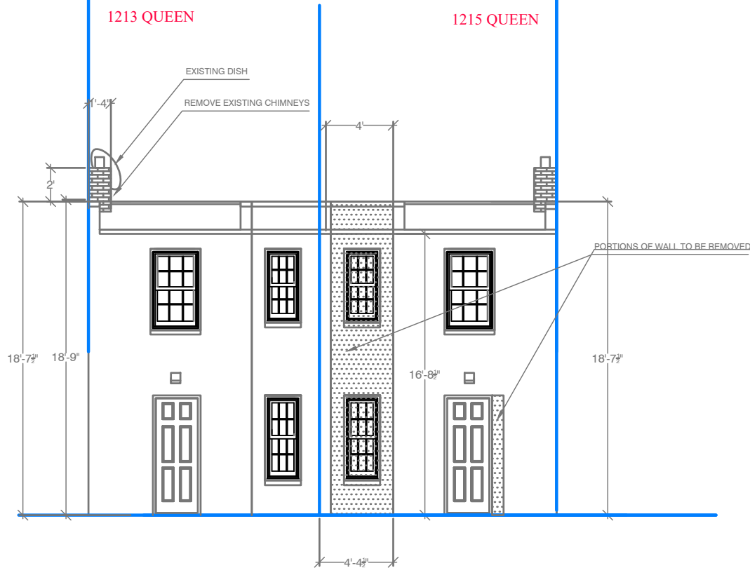
3 EXISTING NORTH ELEVATION A-1 SCALE: 1/8" = 1'-0"
