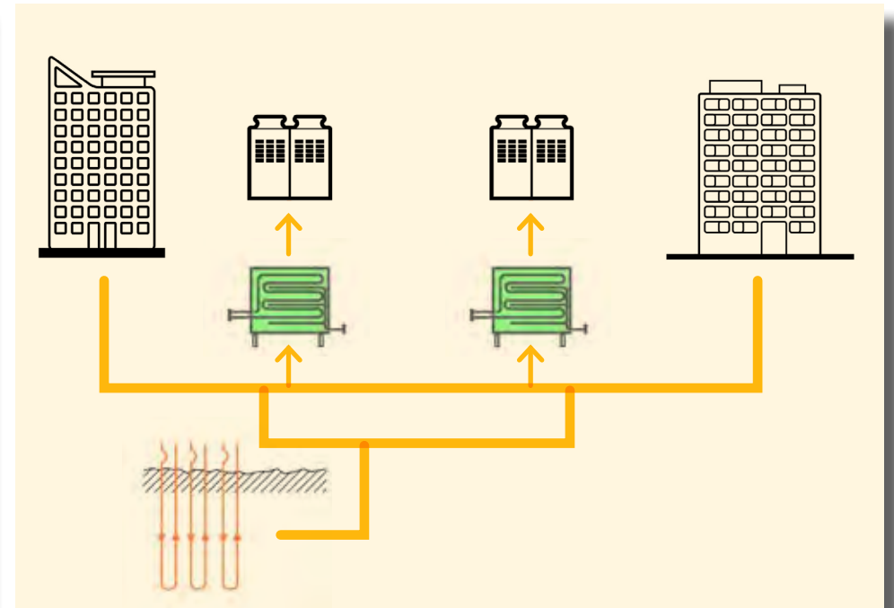
SCENARIO 2: CW + AMBIENT LOOP + GSHP
